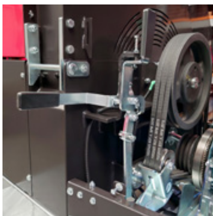
Direkte start. Til- og frakobling af remme.
